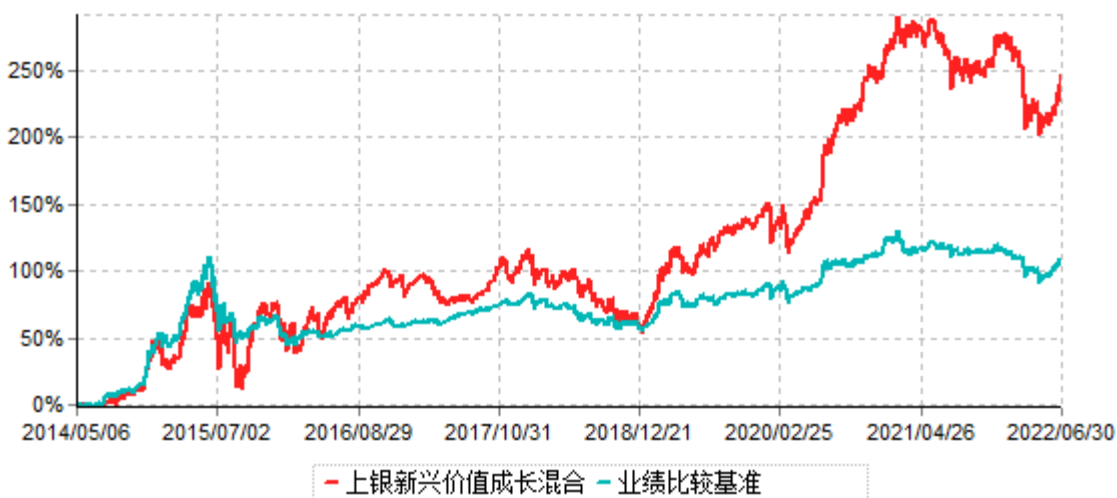
上银新兴价值成长混合型证券投资基金累计净值增长率与业绩比较基准收益率历史走势对比图 (2014年05月06日-2022年06月30日)
